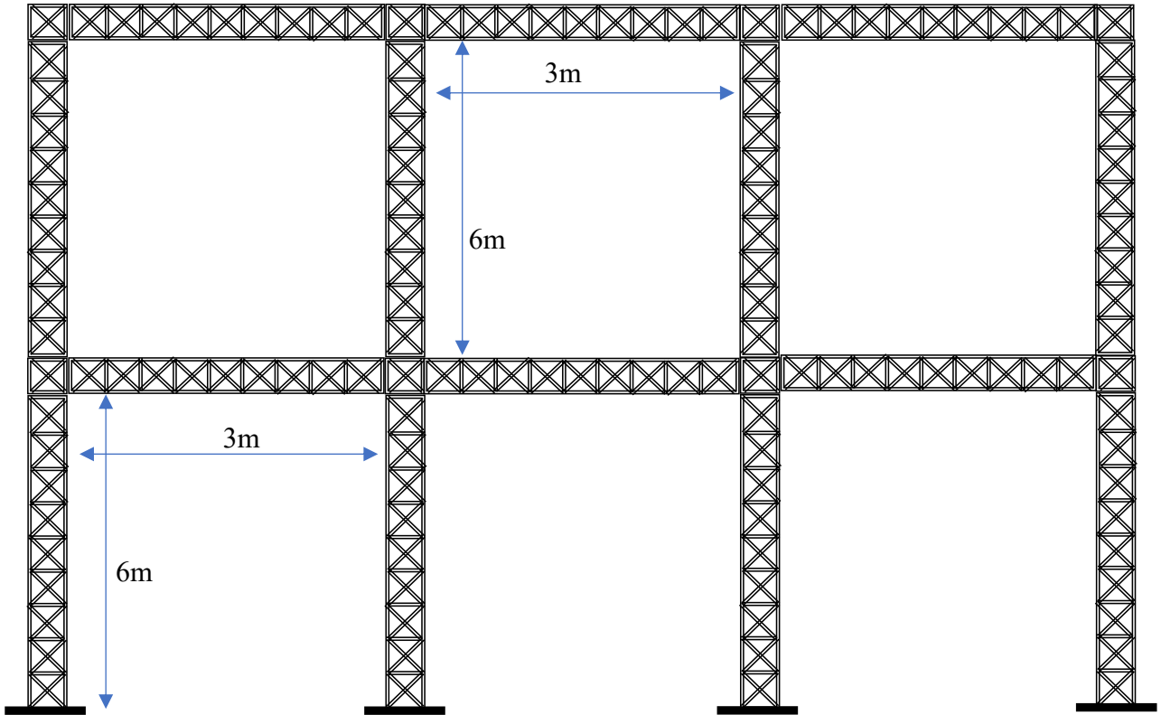
Alçado 1
