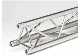
WORKiW WTX 29/100 Color: Aluminio o Negro. Truss triangular de aluminio. 290 mm de lado. 1 m de longitud. Tubo 50 mm.
