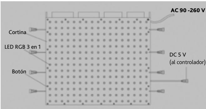
Estructura de la pantalla (Frontal)
