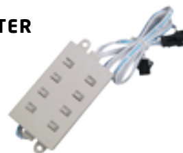
Splitter para el conexionado de hasta 8 lámpara LD5 RGB. Conexiones de entrada y salida para conectar al controlador y a otros LD SPLITTER hasta completar una red de 100 lámparas por puerto.
