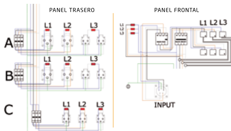
Esquema eléctrico.
