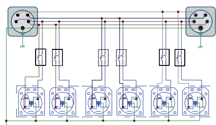
Cableado interno: esquema de conexión (PS 32).
