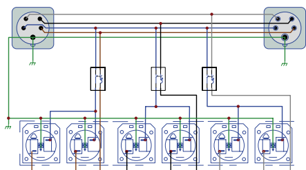
Cableado interno: esquema de conexión (PS 16).
