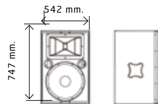
MINO 15 A PRO
