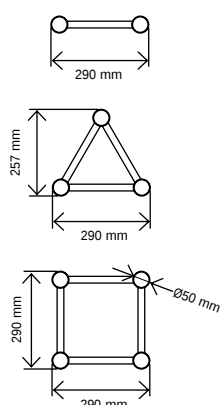
Serie 29 -TRUSS PRO
