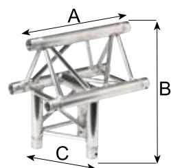
3 LADOS 90° VERTICAL VÉRTICE-T SUPERIOR
