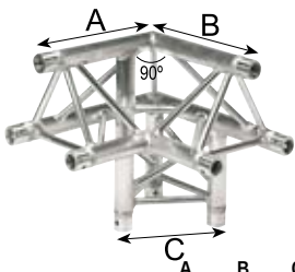
3 LADOS 90° ESQUINA VÉRTICE SUPERIOR DERECHA
