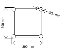
Serie 40 -TRUSS PRO
