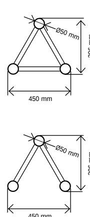
Serie 40 -TRUSS PRO
