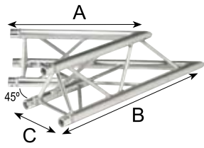
2 LADOS 45° ESQUINA HORIZONTAL
