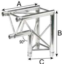
2 LADOS 90° VERTICAL ESQUINA VÉRTICE INFERIOR
