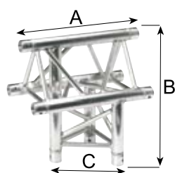
3 LADOS 90° VERTICAL VÉRTICE-T SUPERIOR
