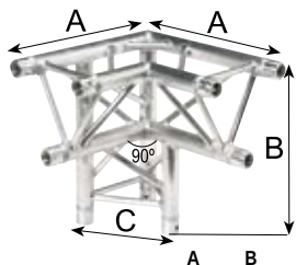
3 LADOS 90° ESQUINA VÉRTICE INFERIOR IZQUIERDA
