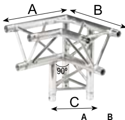
3 LADOS 90° ESQUINA VÉRTICE INFERIOR DERECHA
