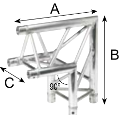
2 LADOS 90° VERTICAL ESQUINA VÉRTICE SUPERIOR
