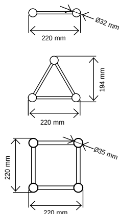
Serie 22 -TRUSS DECO
