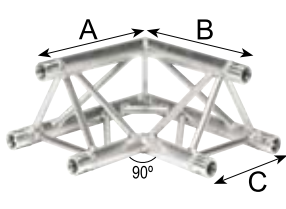
2 LADOS 90° ESQUINA HORIZONTAL
