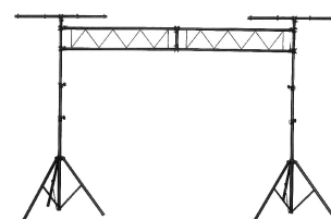
AMS SET PUENTE DISCO MK 3 Estructura para iluminación de escenarios. 300 x 160/322 cm. Aluminio. Negro.
