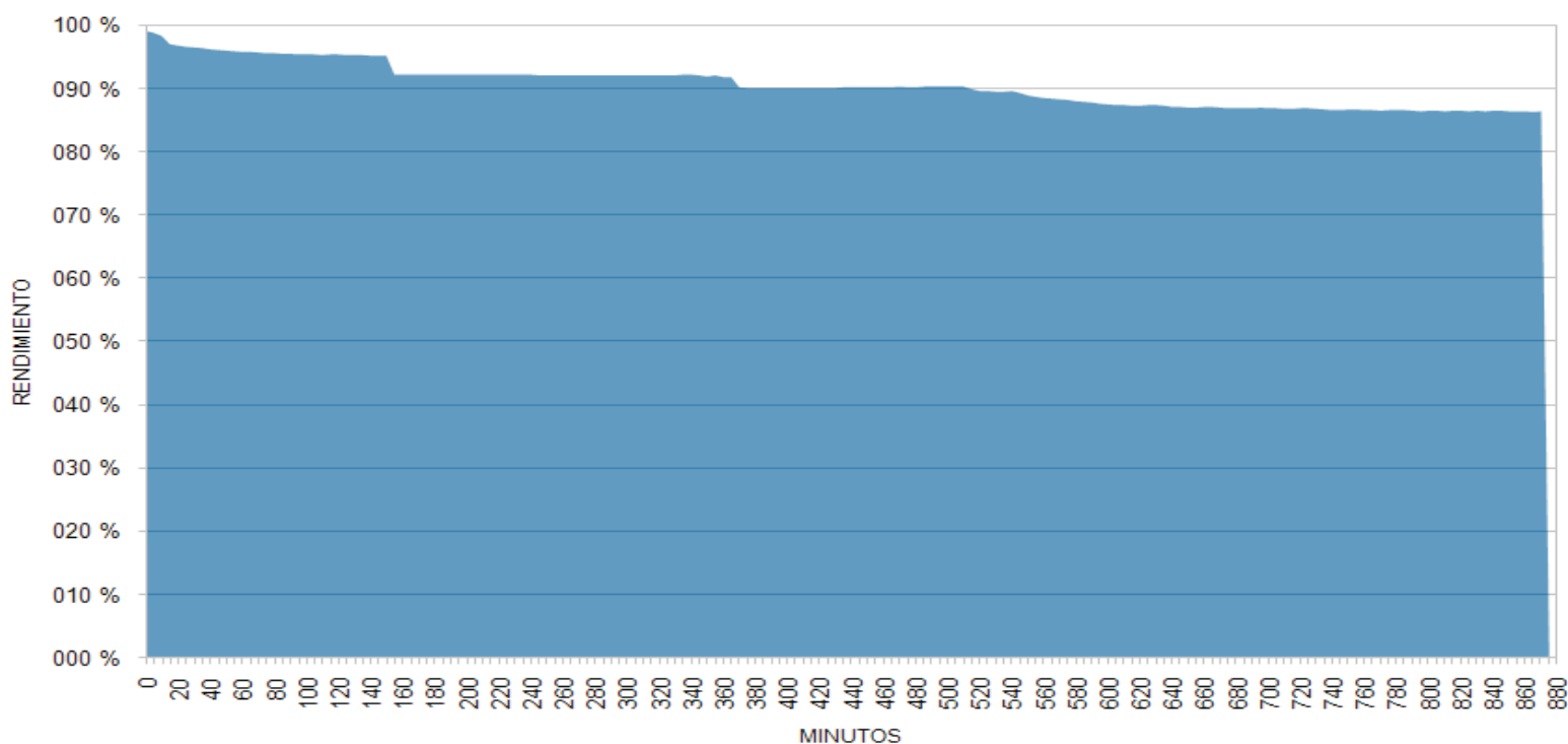
GRÁFICA DESCARGA - SOLO ROJO 100%
