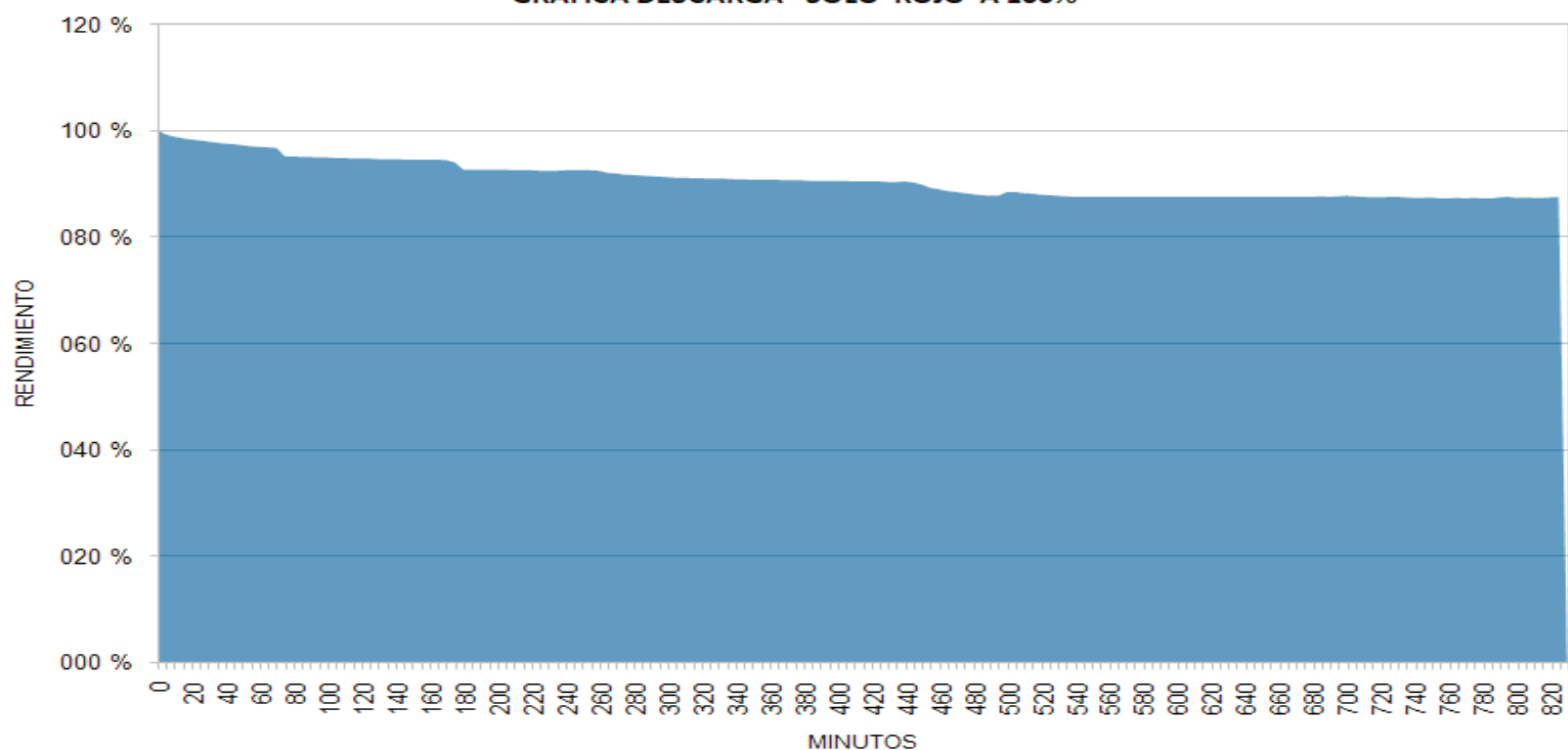
GRÁFICA DESCARGA - SOLO ROJO A 100%
