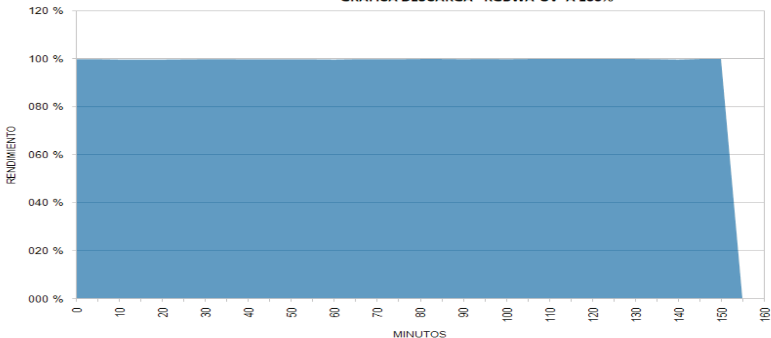
GRÁFICA DESCARGA - RGBWA-UV A 100%
