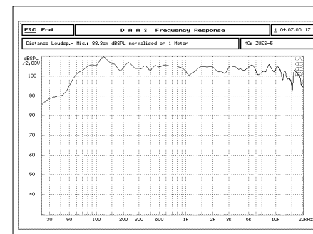
Respuesta de Frecuencia
