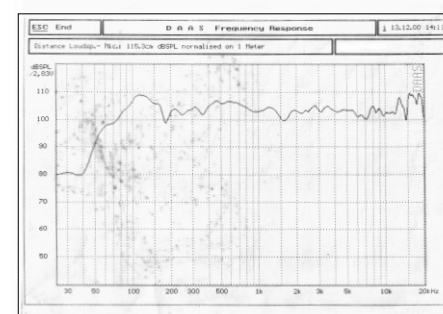
Respuesta de Frecuencia
