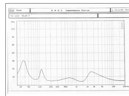
Curva de Impedancia
