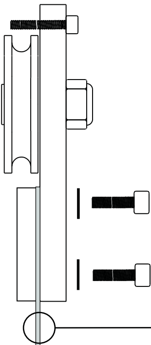
Steel Profile (Section) Perfil de acero (Sección)
