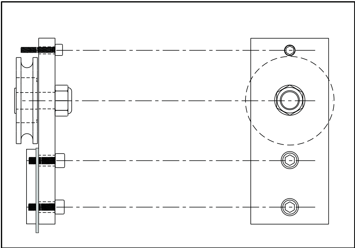
Steel Profile (Section) Perfil de acero (Sección)
